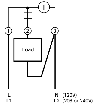
SPST
