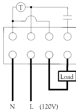
SPST
