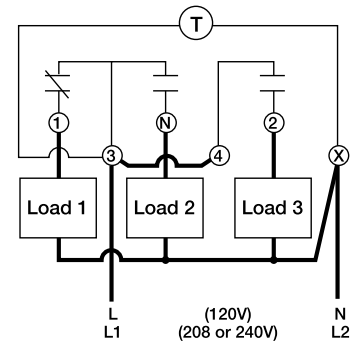
SPST
