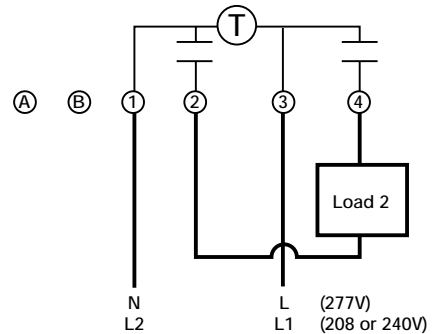
DPST
