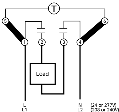
DPST
