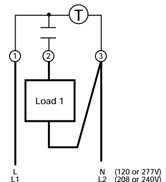
SPST
