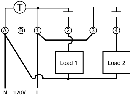
DPST
