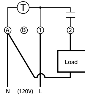
SPST
