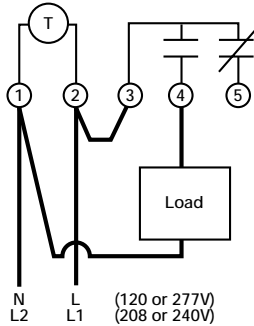
SPDT
